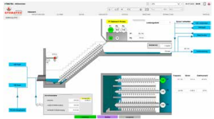
Übersicht einer Teilanlage im Prozessleitsystem
